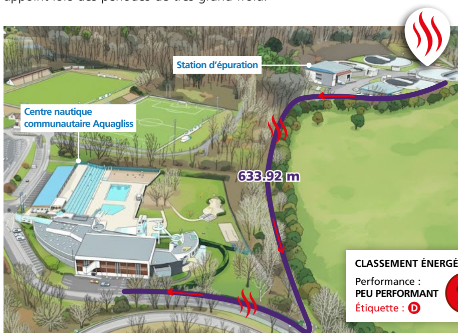
Représentation schématique de la récupération de la chaleur de la station d'épuration pour chauffer l'eau des bassins Aquagliss
